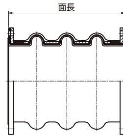
SJ-K200S (偏心量200mm・中圧用)
