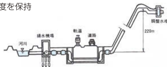
試験圧力 4.4MPa 対応品の設置例
