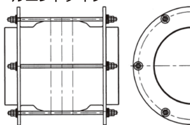
ベベルエンドタイプ
