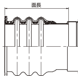
SJ-K200S (偏心量200mm・中圧用)
