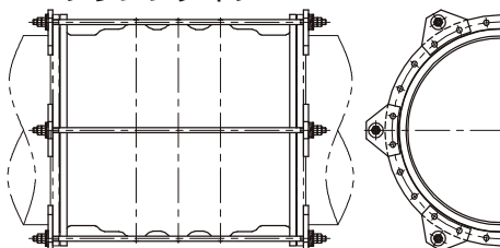
フランジタイプ
